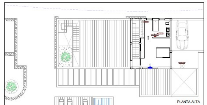
PLANO DE CALIDAD DE AIRE E:1/100
